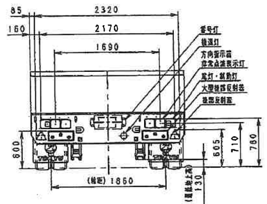
東急 TE28J3E3S型 トレーラ全体図
